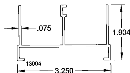
3 FRAME JAMB
